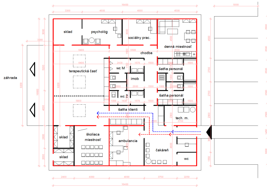
Pôdorys 1np
